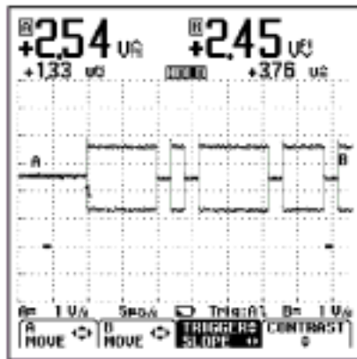
图4. 改变时基，您可以放大并分析信号的细节
