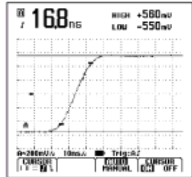
图5. Fluke 124自动测量上升时间
